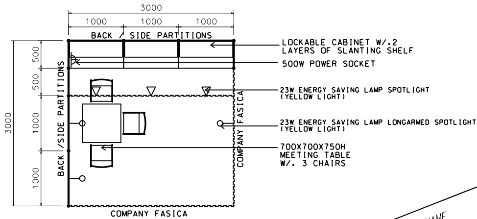
PLAN 平面圖
