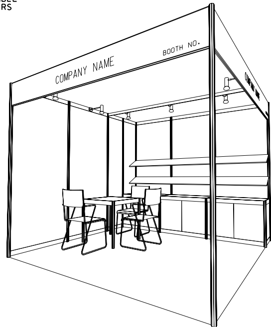
PERSPECTIVE 透視圖
