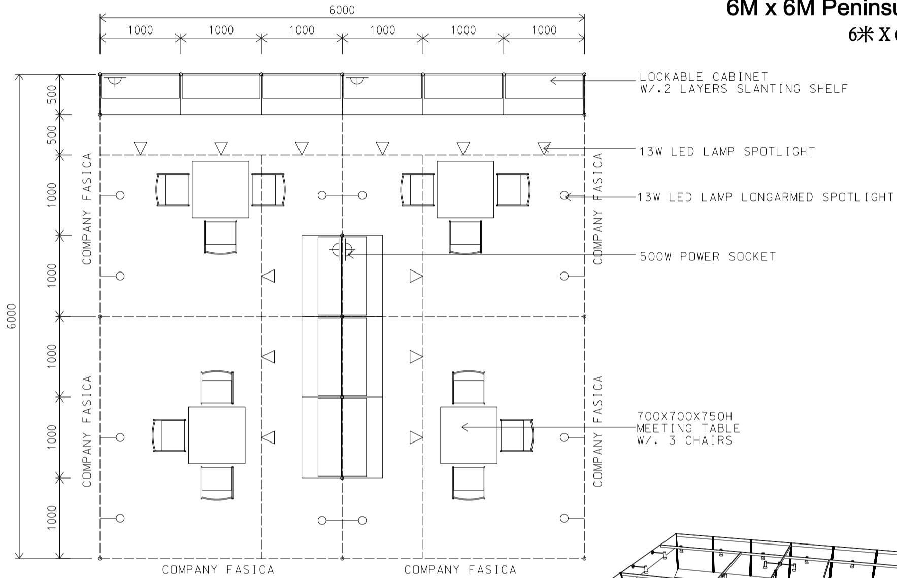
PLAN 平面圖
